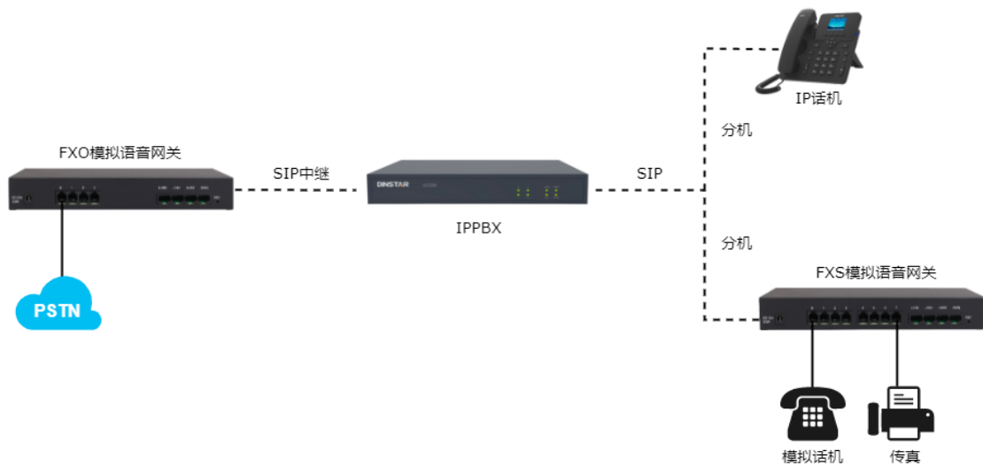
图-应用拓扑图
